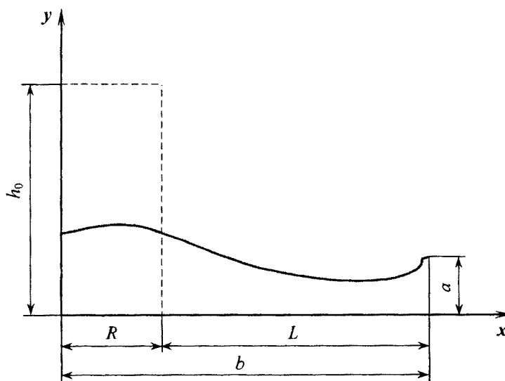
Рис. ПЗ.2. Типичная картина движения жидкости в обваловании при квазимгновенном разрушении резервуара ----- - уровень начального столба жидкости; ————— - уровень жидкости в промежуточный момент времени (результаты расчета)
